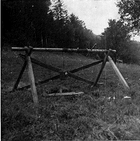
Abb. 10 Brunnwinde
