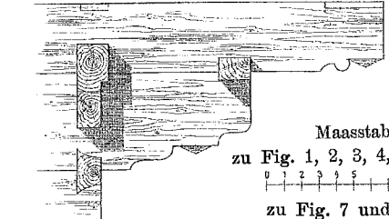
Fig. 6. Seitenansicht der Endpfette und Endconsole.
