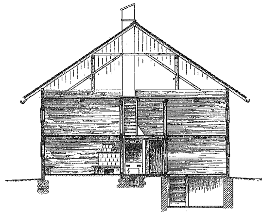
Schnitt S S.
