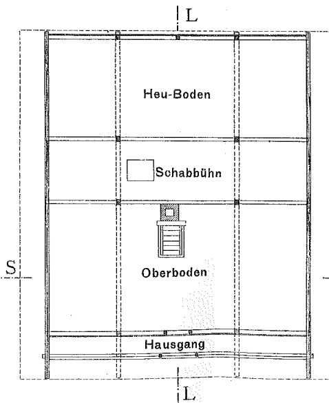
Dachboden.
