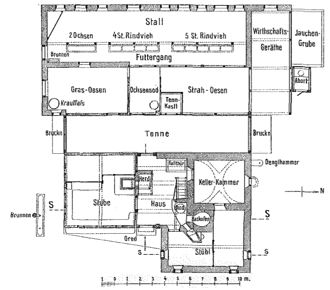
Ebenerd-Geschoss.
