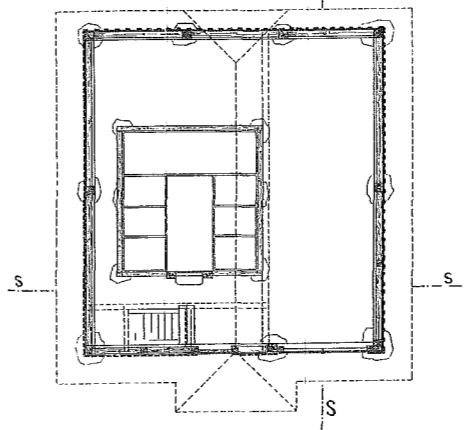
Grundriss.
