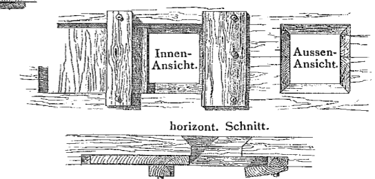
Fig. 7. Fenster der Rauchkammer.
