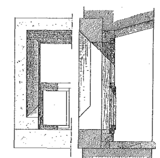
Fig. 7. Fenster der Rauchkammer.
