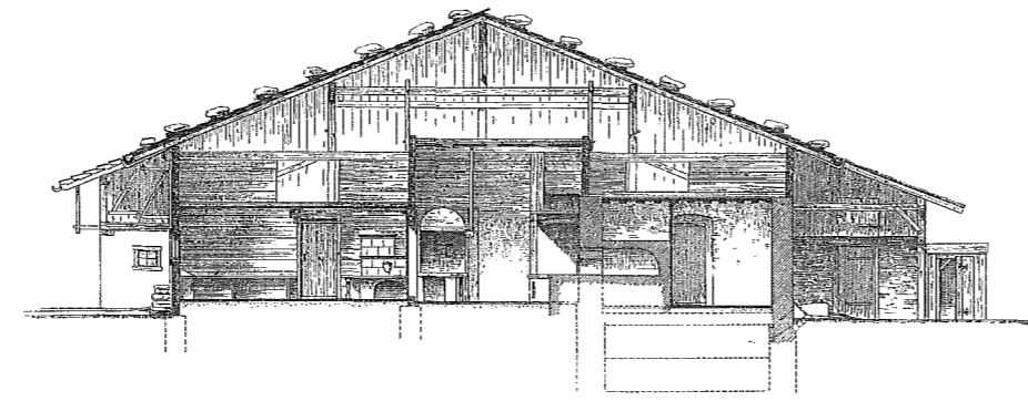
Querschnitt ss.
