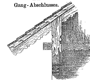
Fig. 3. Querprofil. (Schnitt P P.) mit Seitenansicht der Gangeconsole.
