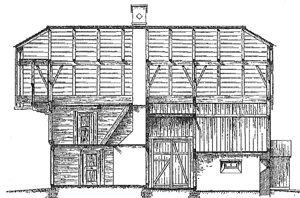
Schnitt L L.
