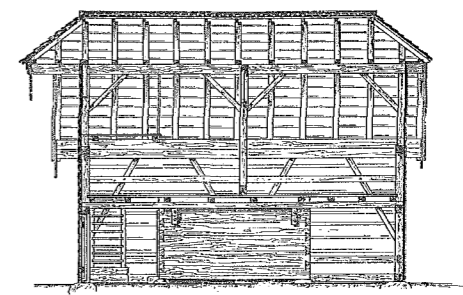
Längsschnitt ss.
